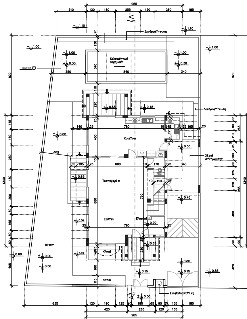
ΚΑΤΟΨΗ ΙΣΟΓΕΙΟΥ / Ground Floor Plan
