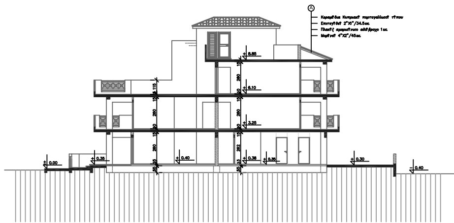
TOMH A - A' SECTION A - A'
