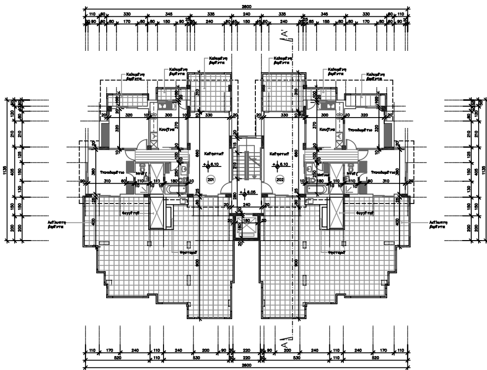
ΚΑΤΟΠΗ Β' ΟΡΟΦΟΥ / SECOND FLOOR PLAN
