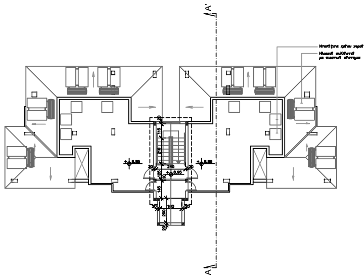
ΚΑΤΩΦΗ ΤΑΡΑΤΣΑΣ ROOF PLAN
